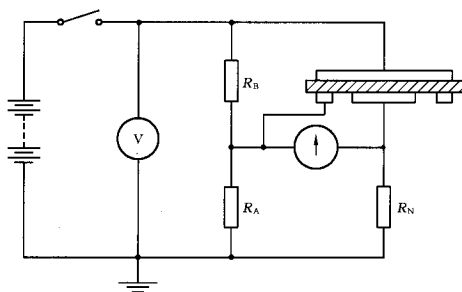
图 6 用于测量体积电阻的惠斯登电桥法
